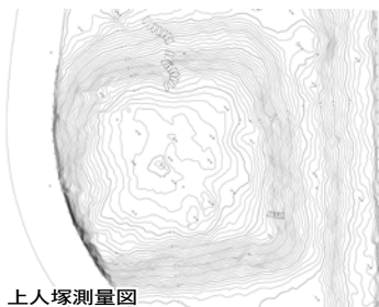
上人塚測量図
