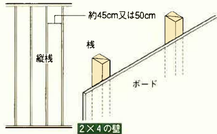
2×4の壁
