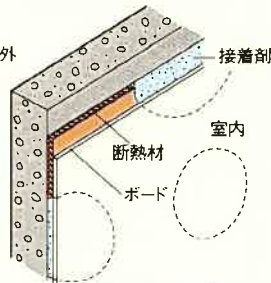
GL工法防露壁
