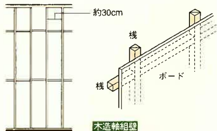
木造軸組壁
