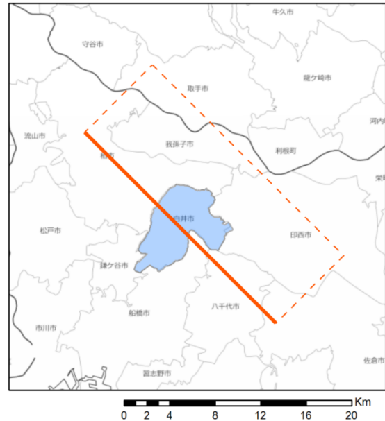
想定震源断層の位置
