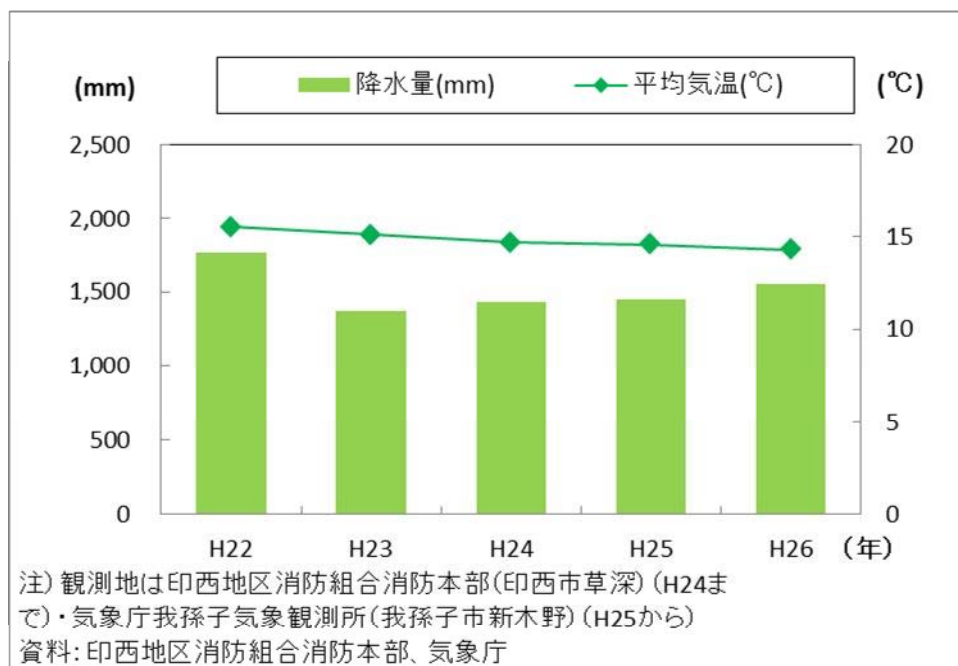
図2-1-2 市の気象
