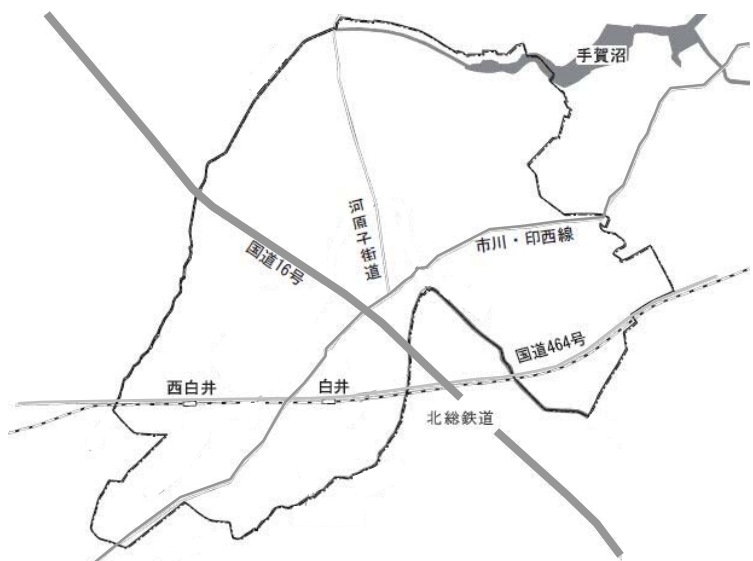
図2-1-6 市の交通網
