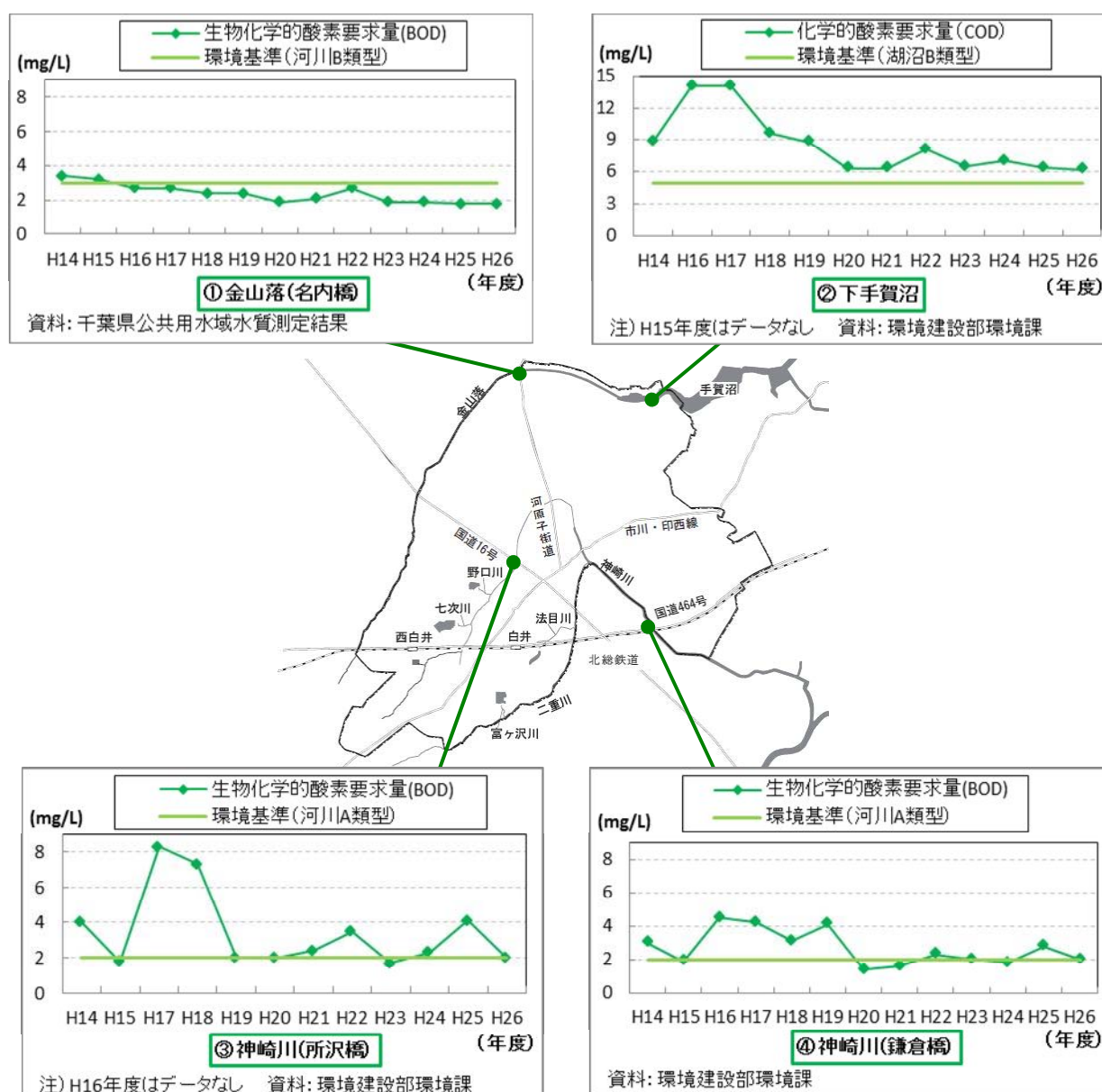
図2-3-2 河川・湖沼の水質状況
