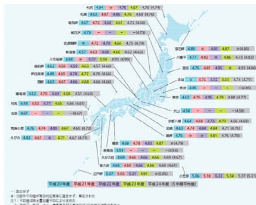
図2-7-3 降水中の pH の推移
