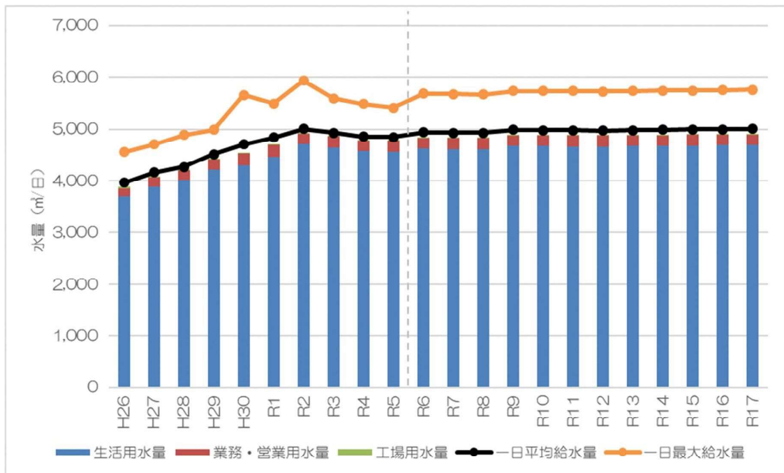
図 4-2 給水量の将来見通し
