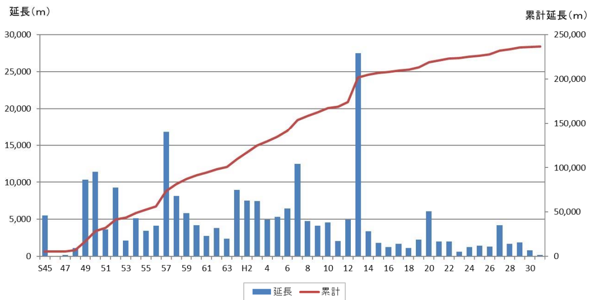
図3-12 布設年度別の管きよ延長
