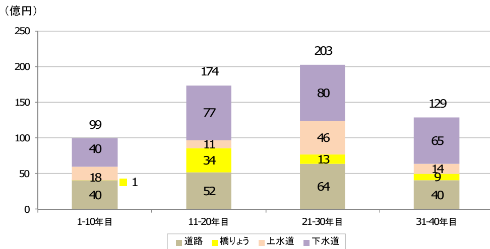
図3-30 土木系公共施設の更新費用
