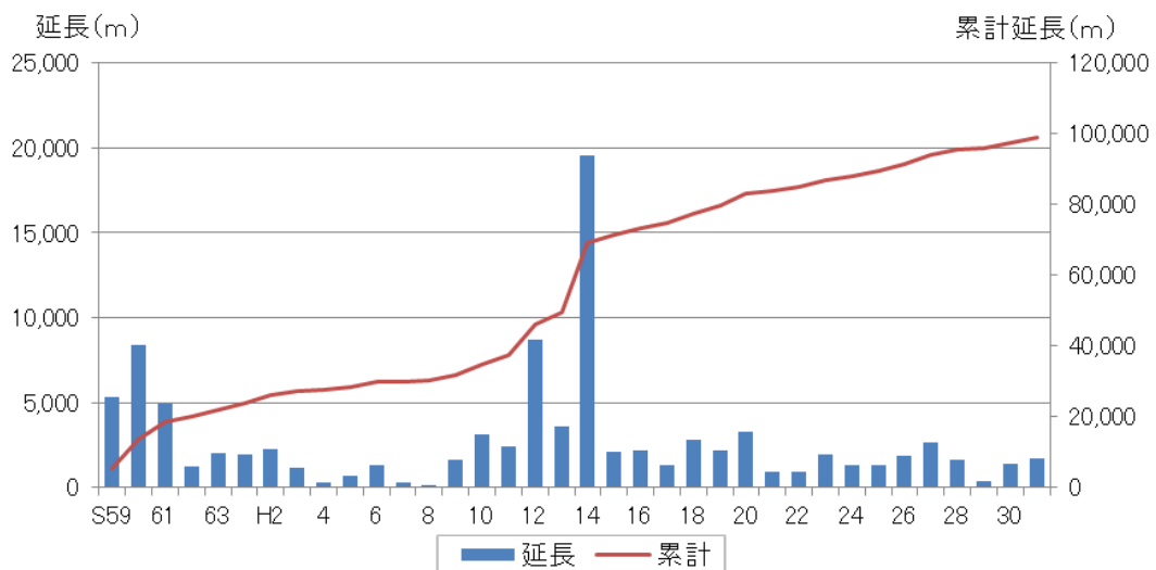
図3-10 布設年度別の配水管延長
