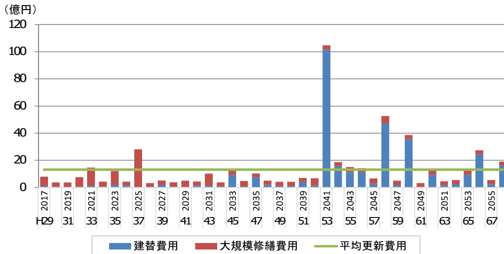
図3-28 建築系公共施設の更新費用
